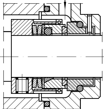
NV-3.2 karbid silicijuma, utisnut u rotirajući prsten
