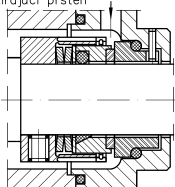
NV-3.3 Karbid volframa, ulemeljen u rotirajući prsten
