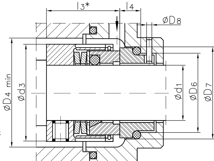
NV-3.1 Karbon grafit, utisnut u rotirajući prsten
